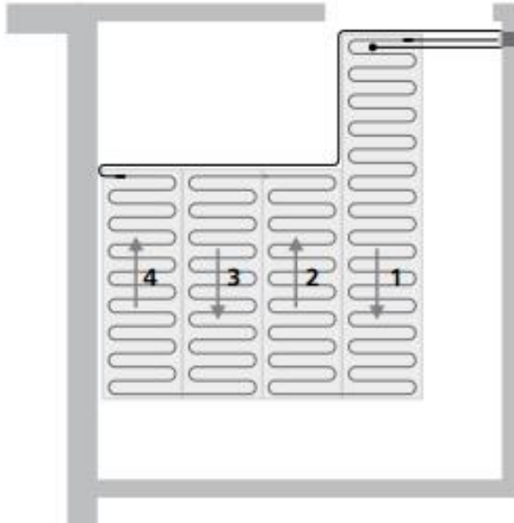
Példa: fűtőszőnyeg konyhai elhelyezése
