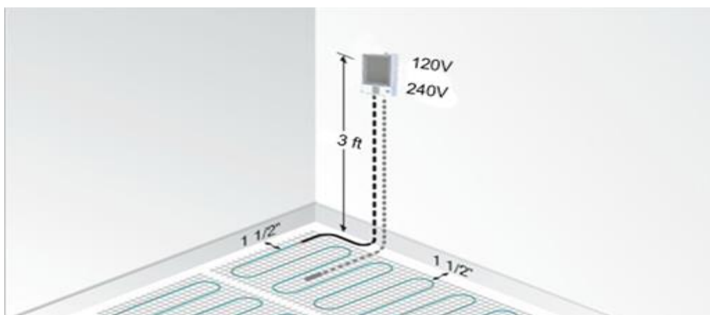
3. Ábra bekötési rajz
